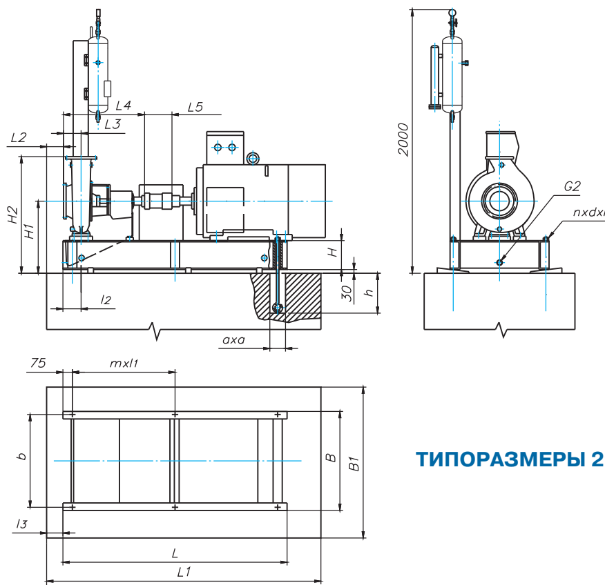
ТИПОРАЗМЕРЫ 2-4, 6-9, 11-14, 16-23, 26, 37
